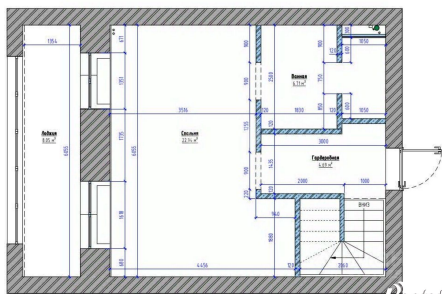
ПЛАН-СХЕМА КОМНАТЫ. 2 ЭТАЖ. 1:45
