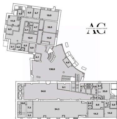
1 этаж
